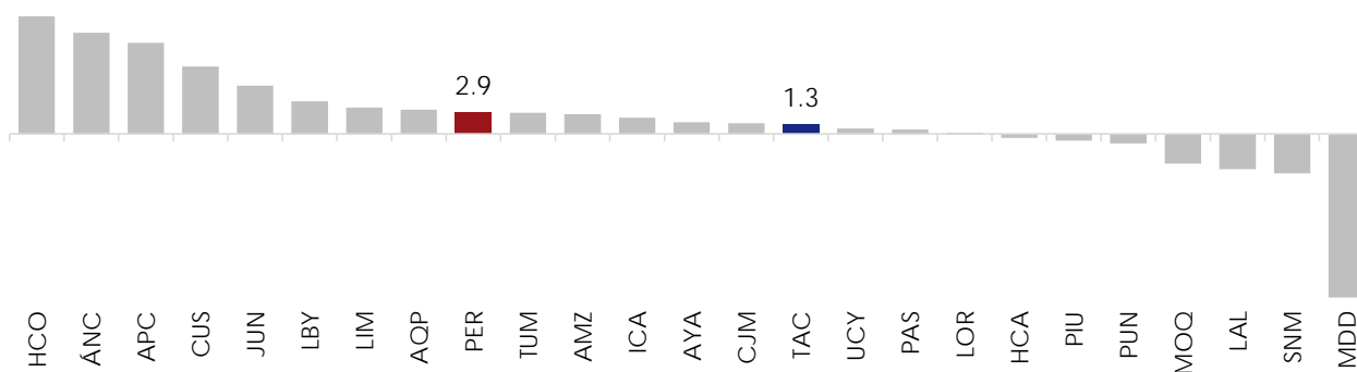
Gráfico 2. Resultados* del ICAE según regiones, 3T-2015
