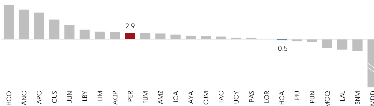
Gráfico 2. Resultados* del ICAE según regiones, 3T-2015
